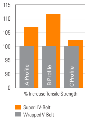
Tensile Strength
