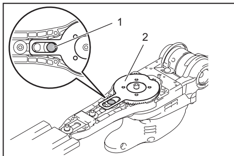
► 1. Protrusion 2. Plate
